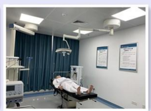
模拟手术室
